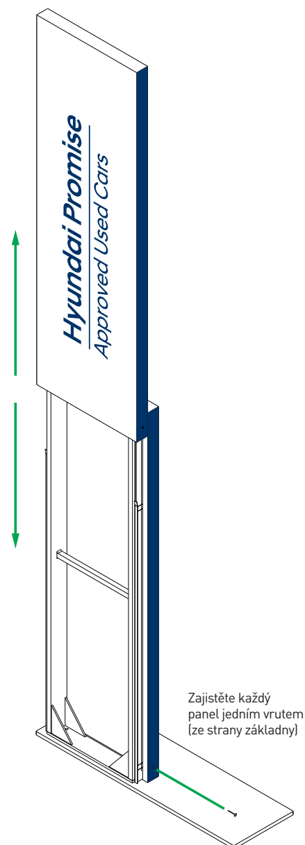
Demontáž/montáž panelů s grafikou
